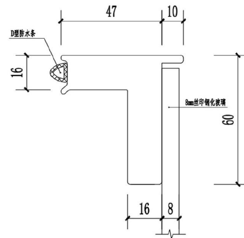
成品门框型材A 1:2
