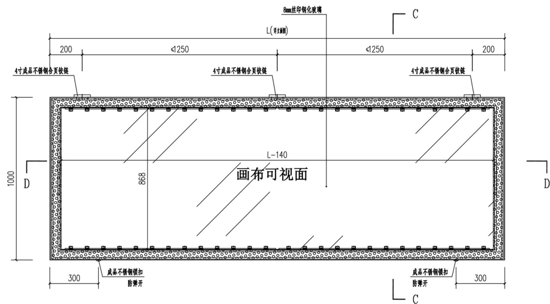
广告灯箱正立面图一 1:10
