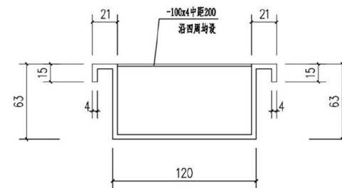
成品门框型材B 1:2
