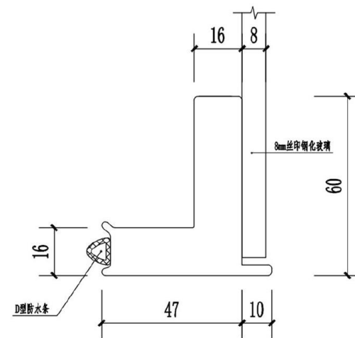
成品门框型材B 1:2
