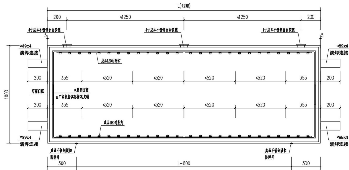
广告灯箱正立面图二 1:10
