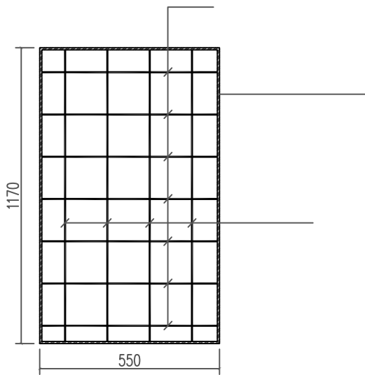
单块预制盖板做法
