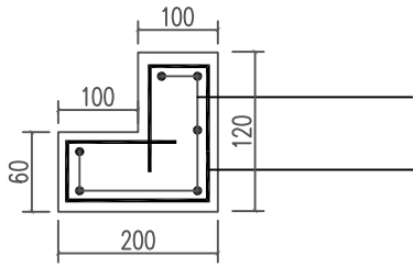
盖座节点A做法
