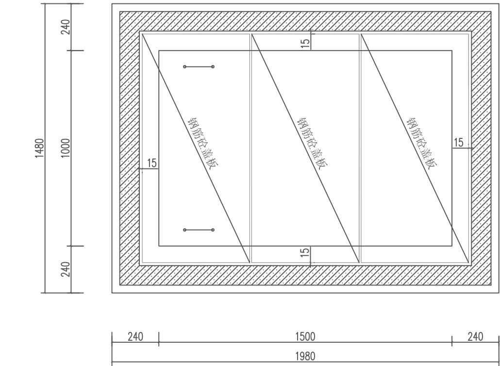
水表井外部平面图
