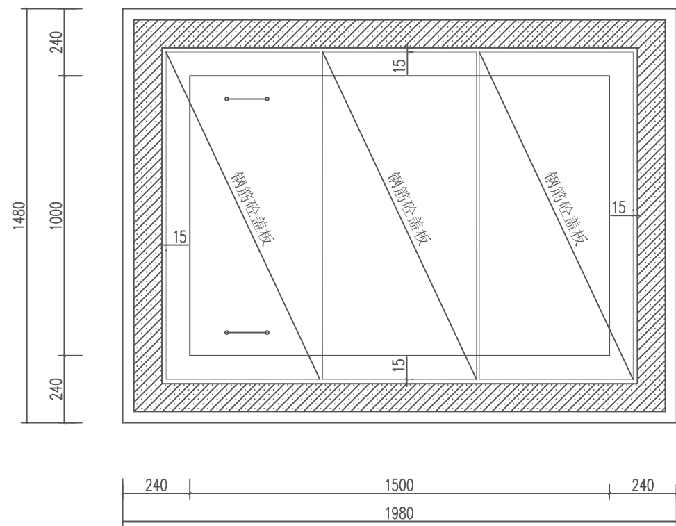
水表井外部平面图
