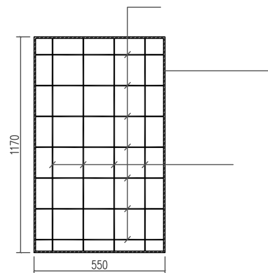
单块预制盖板做法
